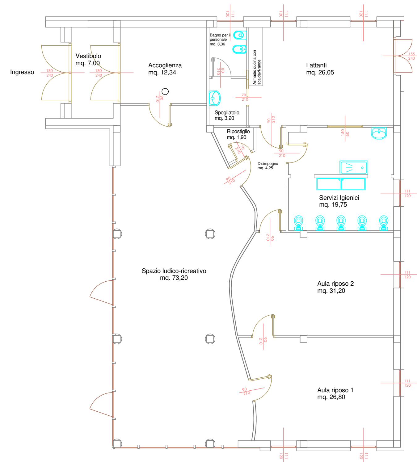
PLANIMETRIA LOCALI ASILO NIDO
